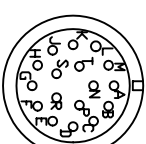
Encoder 신호 PIN 번호 Encoder 신호 PIN 번호 A A U L \bar{A} B V M B C V N \bar{B} D W P Z E W R Z F W R 0V G SHIELD J +5V H
